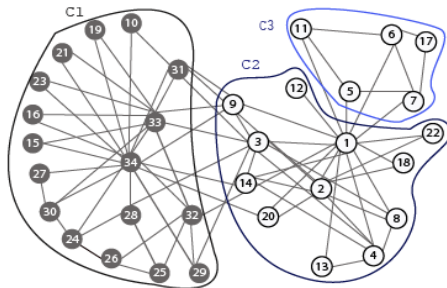
FIGURE 2 – (a) Partition de S1 avec ADV
